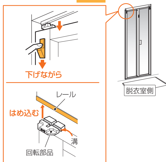
可動側
