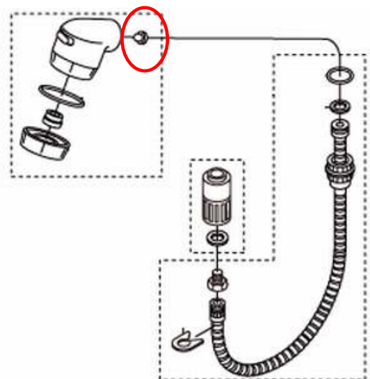
この部品が使われている水栓金具
