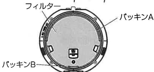
フィルター取り付け状態
