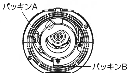
パッキン貼り付け位置
