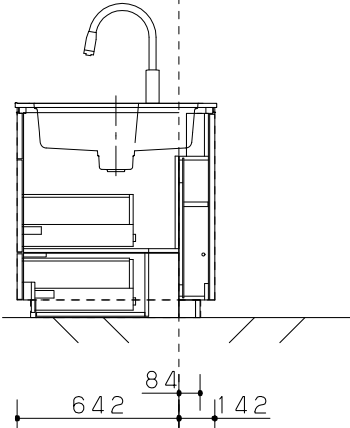
シンク断面
