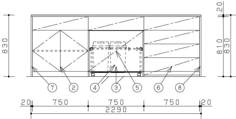
展開図
