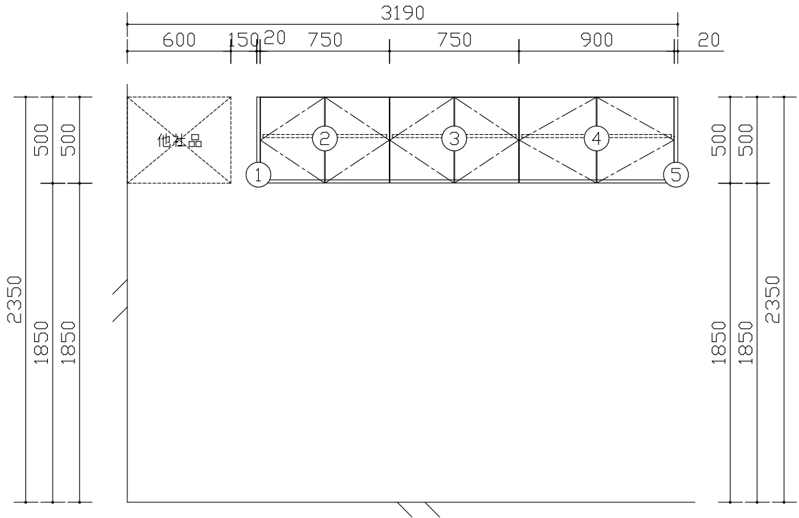
展開図
