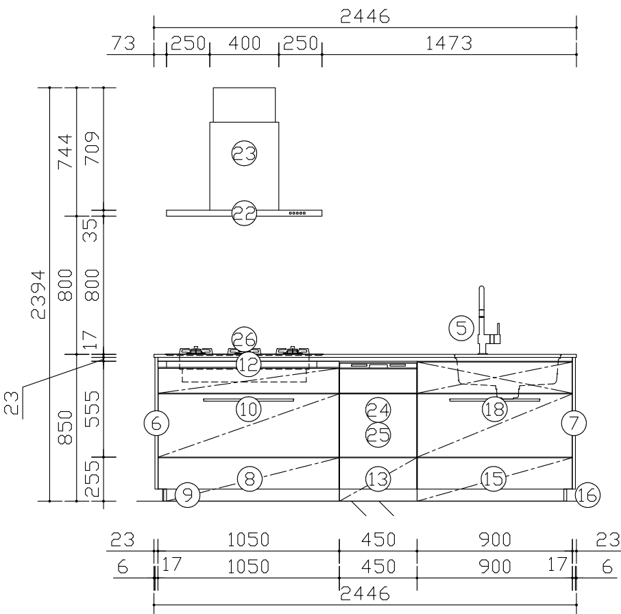
展開図
