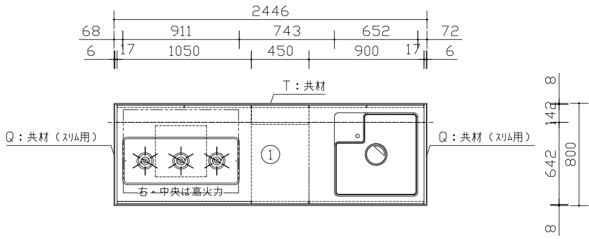
平面図
