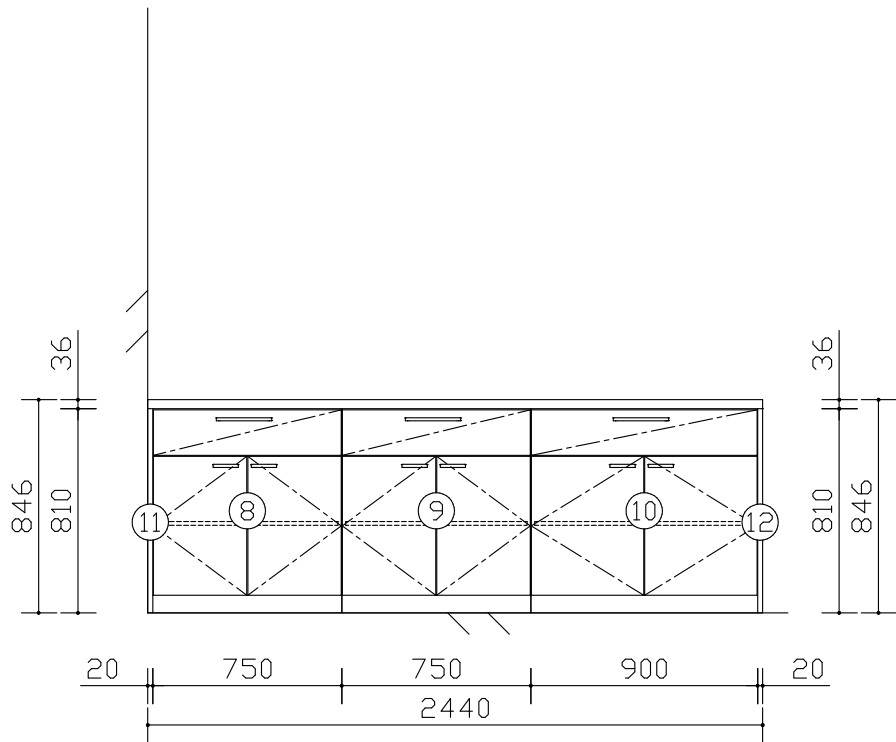
展開図
