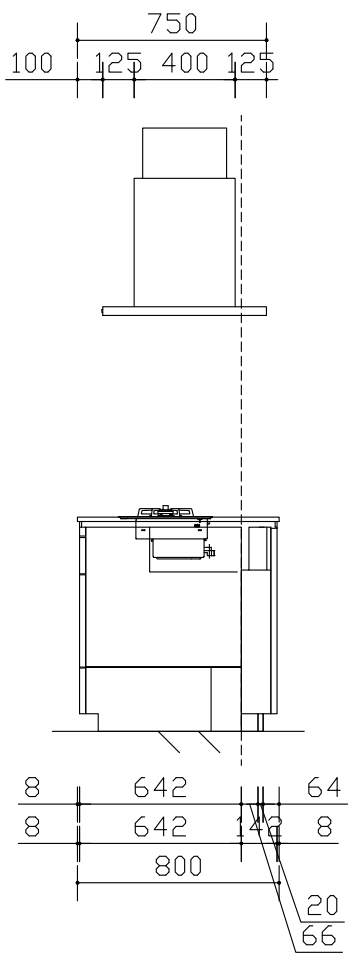
加熱機器断面
