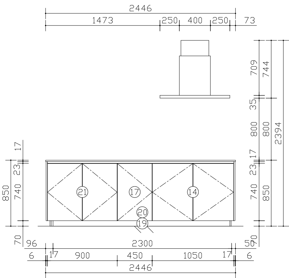
ダイニング側展開図
