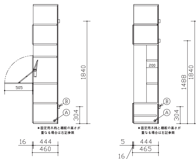
断面図
