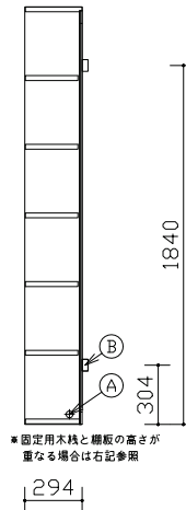
断面図
