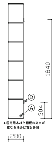
断面図
