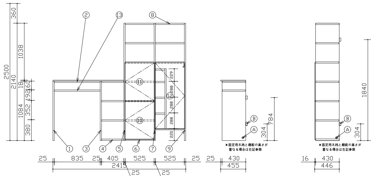
断面図
