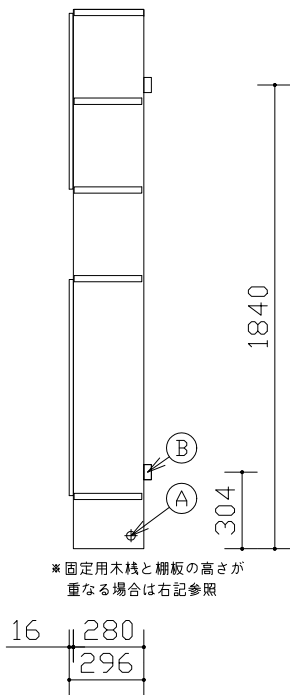
断面図
