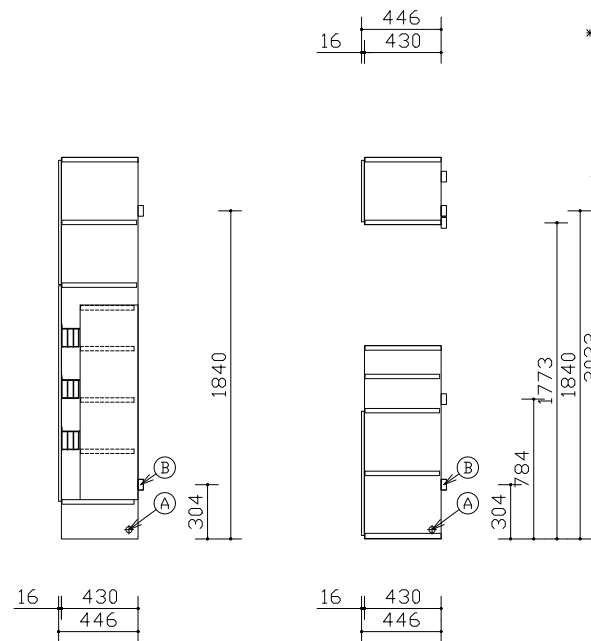
断面図
