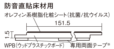
■断面図(mm)
