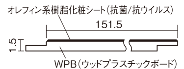
■断面図(mm)
