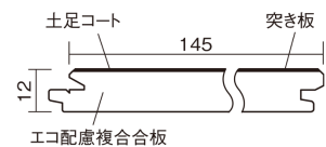
■断面図(mm)
