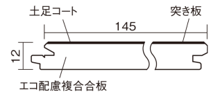
■断面図(mm)
