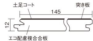
■断面図(mm)
