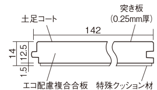
■断面図(mm)
