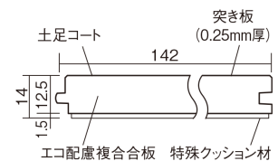
■断面図(mm)
