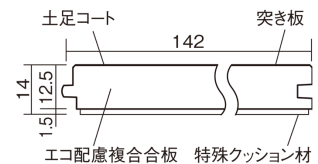
■断面図(mm)
