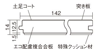
■断面図(mm)
