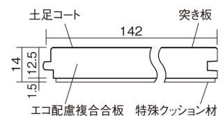
■断面図(mm)
