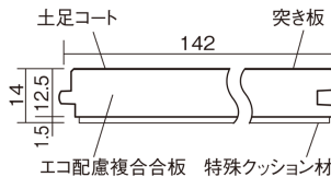
■断面図(mm)
