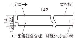
■断面図(mm)
