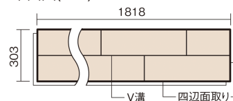
■平面図(mm)
