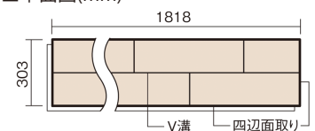
■平面図(mm)
