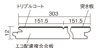
■断面図(mm)
