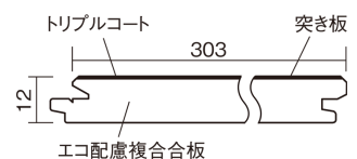
■断面図(mm)
