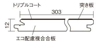
■断面図(mm)
