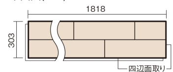
■平面図(mm)
