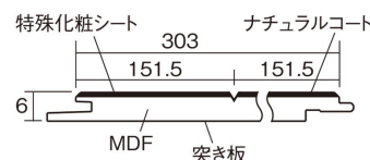
■断面図(mm)
