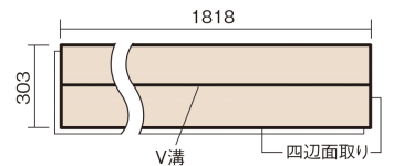
■平面図(mm)
