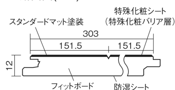
■断面図(mm)
