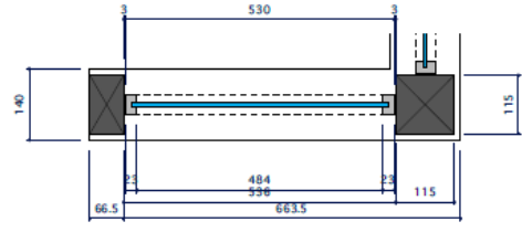
[平面詳細図] S=1/10
