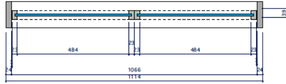
[平面詳細図] S=1/10
