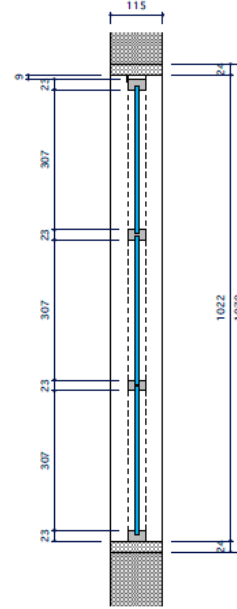
[断面詳細図] S=1/10
