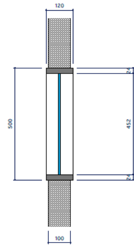
[断面詳細図] S=1/10
