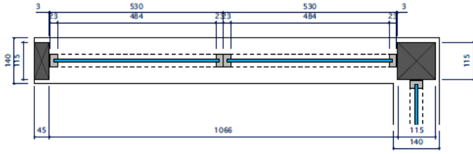
[平面詳細図] S=1/10
