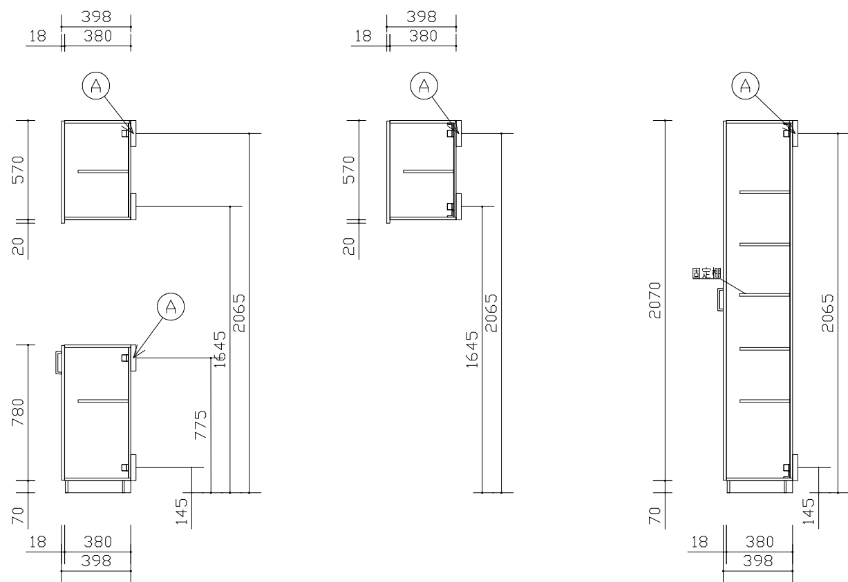
LDK キッチン収納図
