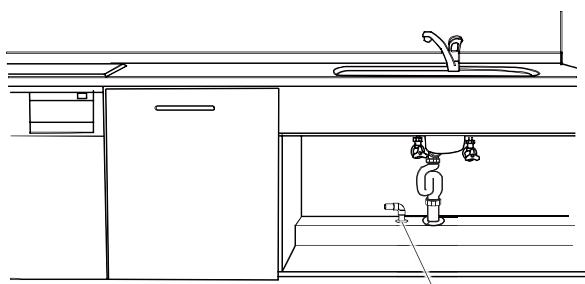
既設配管(HT20)
