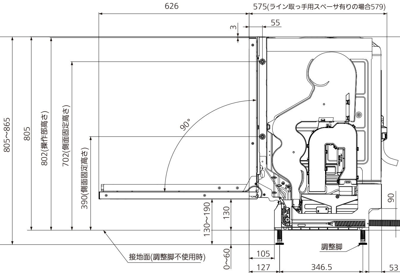
右側面図
