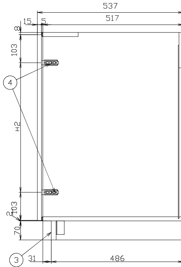
A-A断面図
