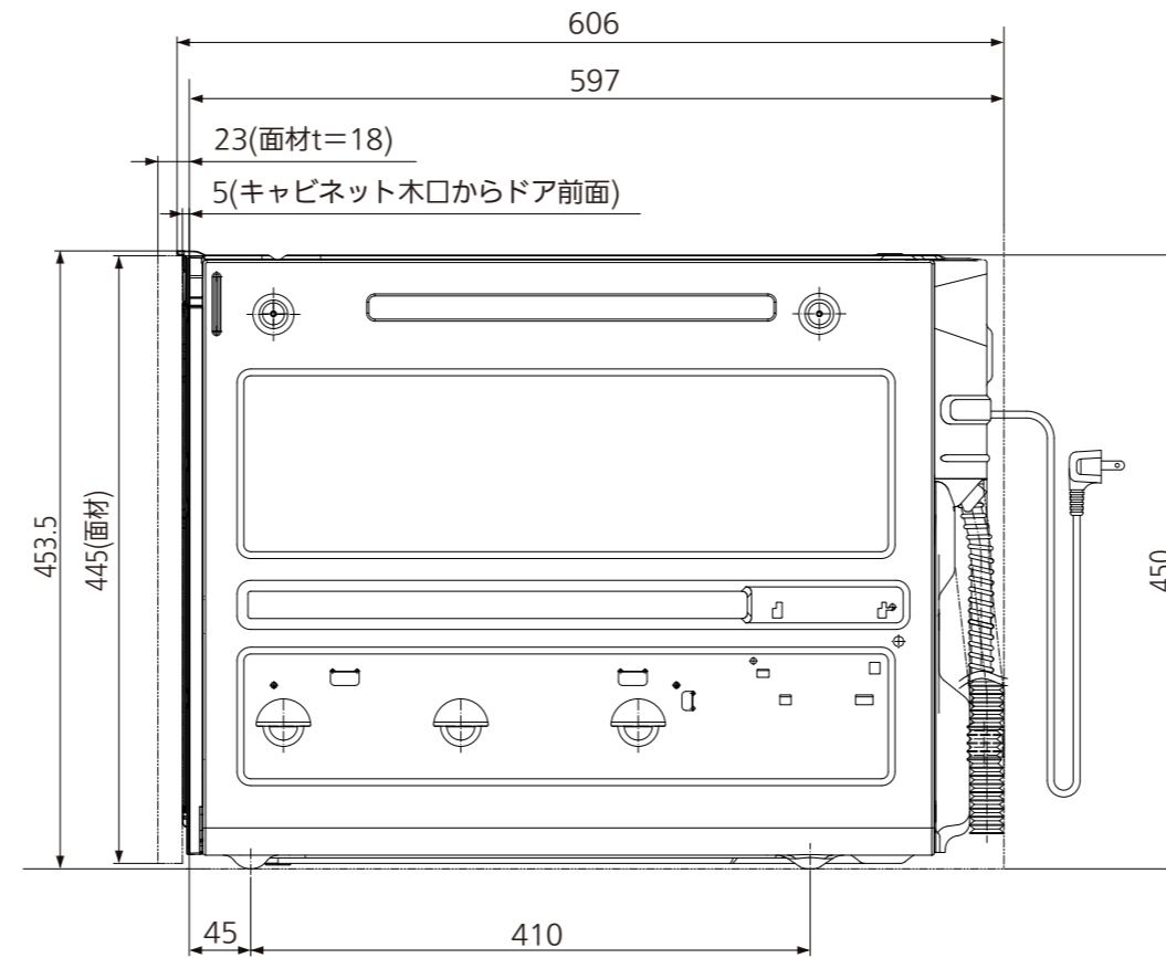
側面図
