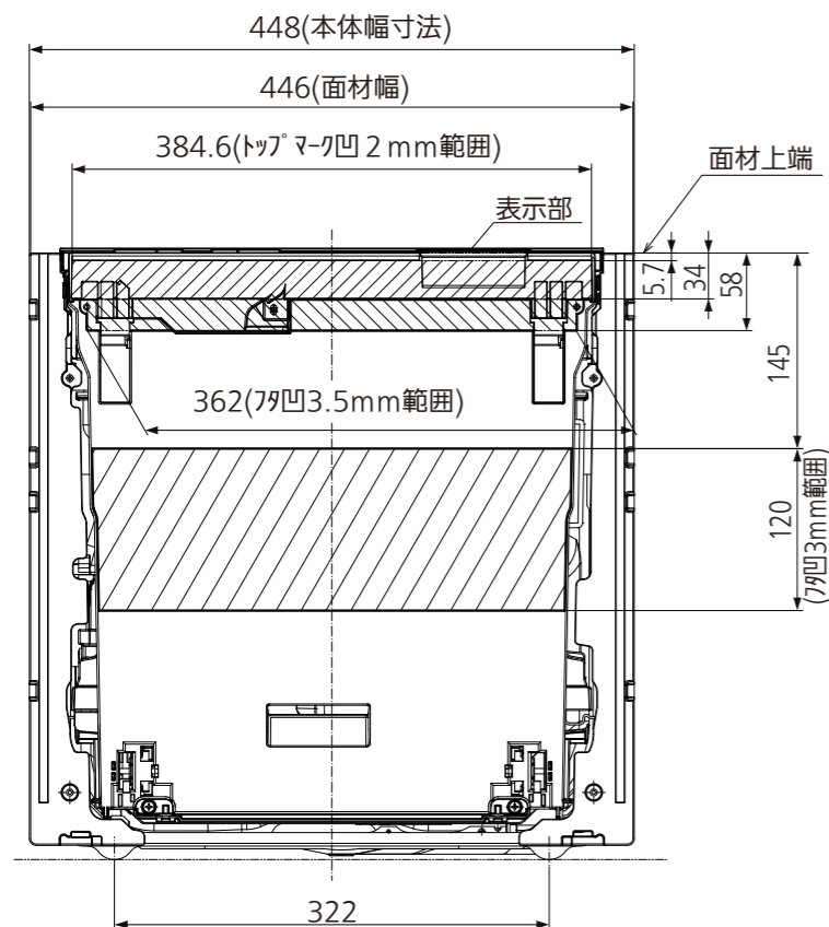
正面図
