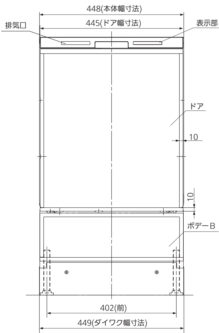
正面図
