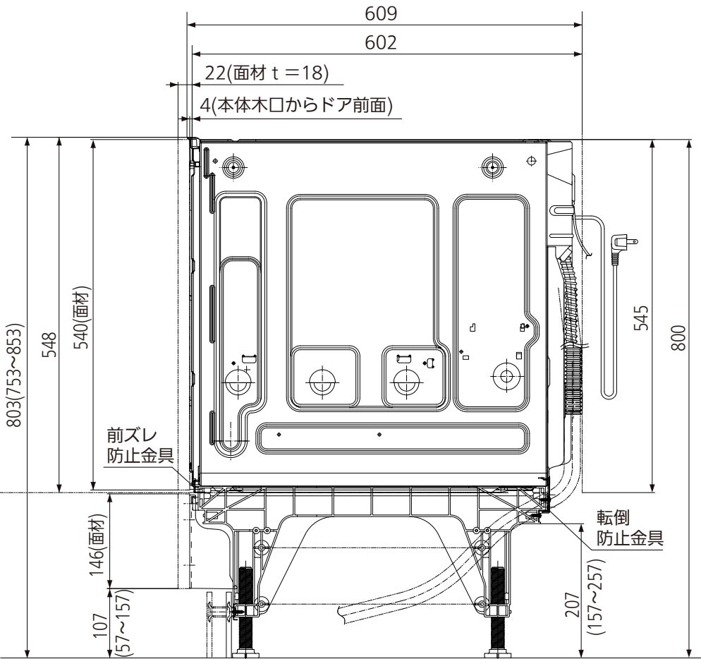
側面図
