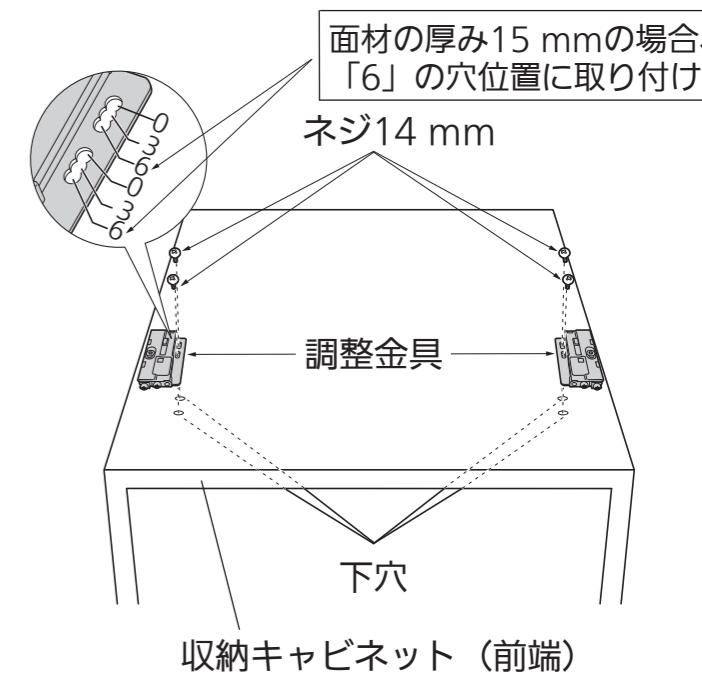
【図3】取り付け事例 (面材の厚み15 mmの場合)
