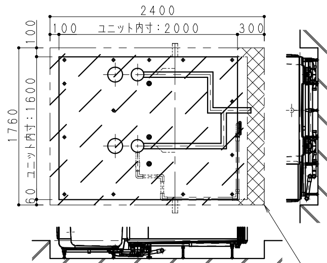
BR勝手ピット設置寸法
