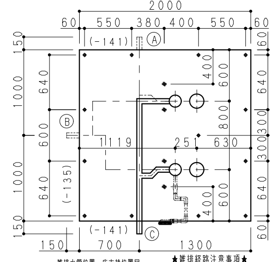
★雑排水経路注意事項★ 排水方向により排水管部材構成内容が変わります。 本図は排水管セットCが同梱されます。
