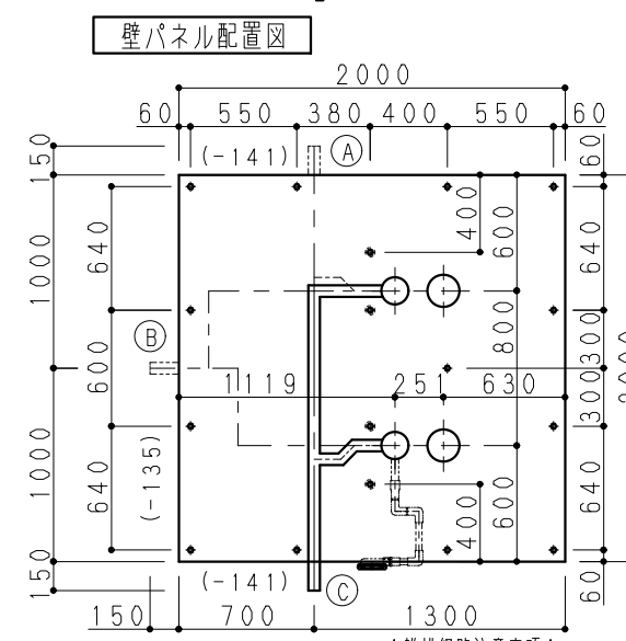
雑排水管位置・床支持位置図 ( ) 寸法はUBFLからの寸法です。 ★雑排水経路注意事項★ 排水方向により排水管部材構成内容が変わります。 本図は配水管セットCが同梱されます。
