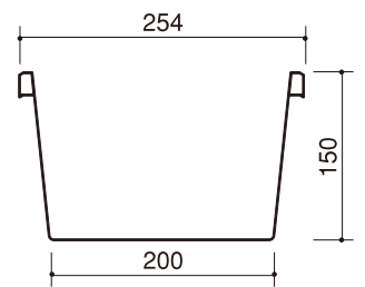
折版200 I 型
