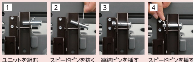
1 ユニットの組む 2 スピードピンを抜く 3 連結ピンを挿す 4 スピードピンを挿す
