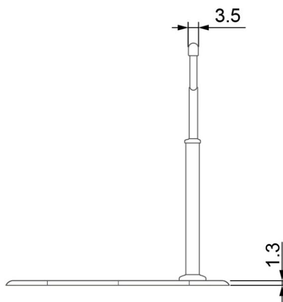
側面図
