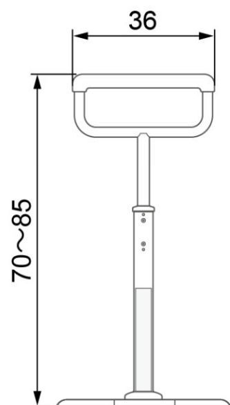
正面図
