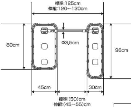
上面図(片手すり)
