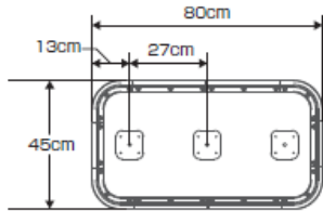
PN-L80601 標準ベース
