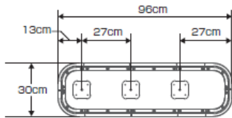
PN-L80602 ステップベース
