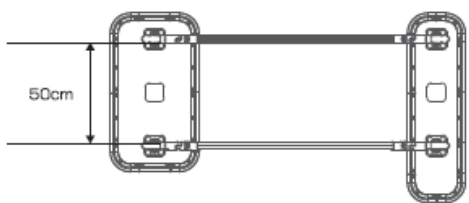
上面図(両手すり)
