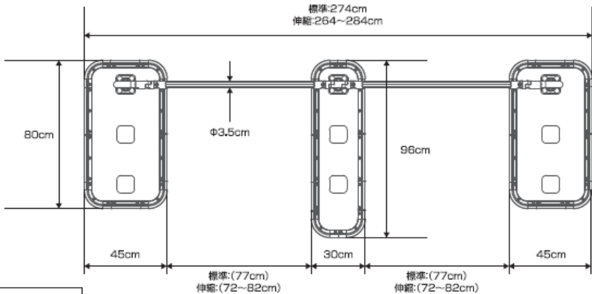
側面図
