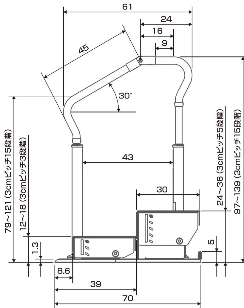
側面図
