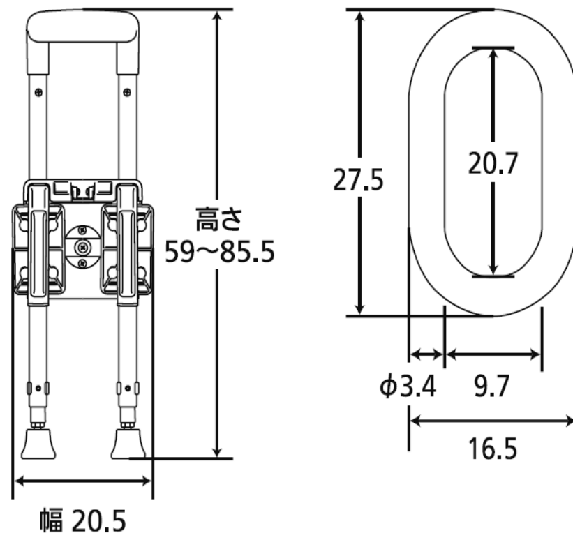
ハンドルの寸法図
