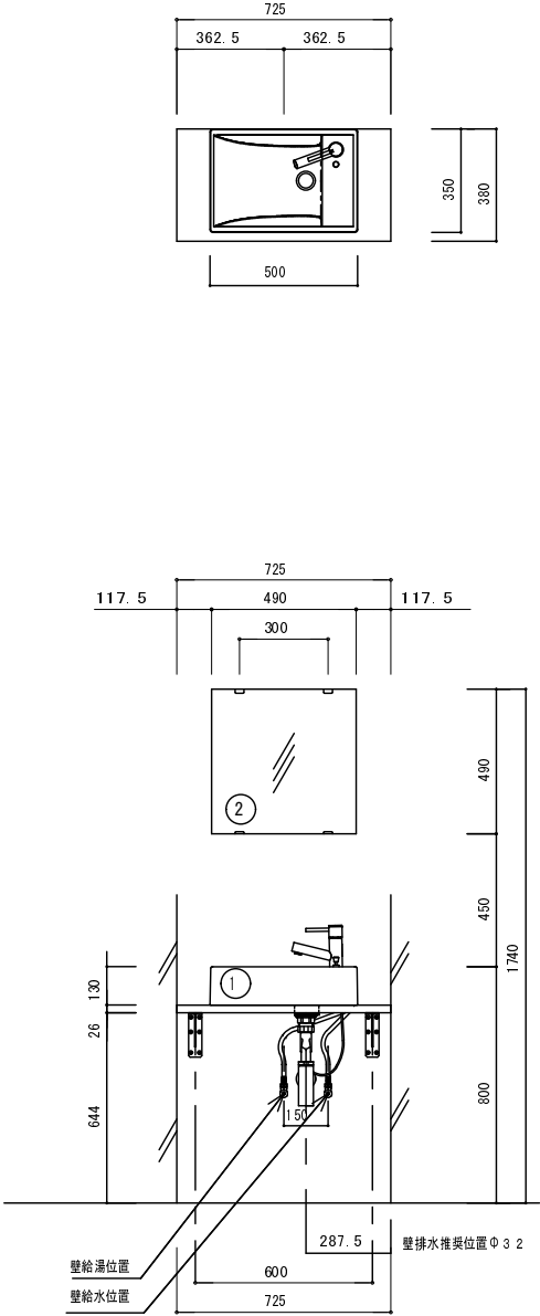
展開図
