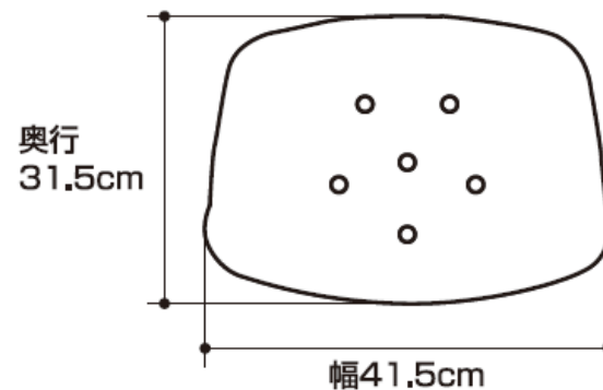
座面寸法図
